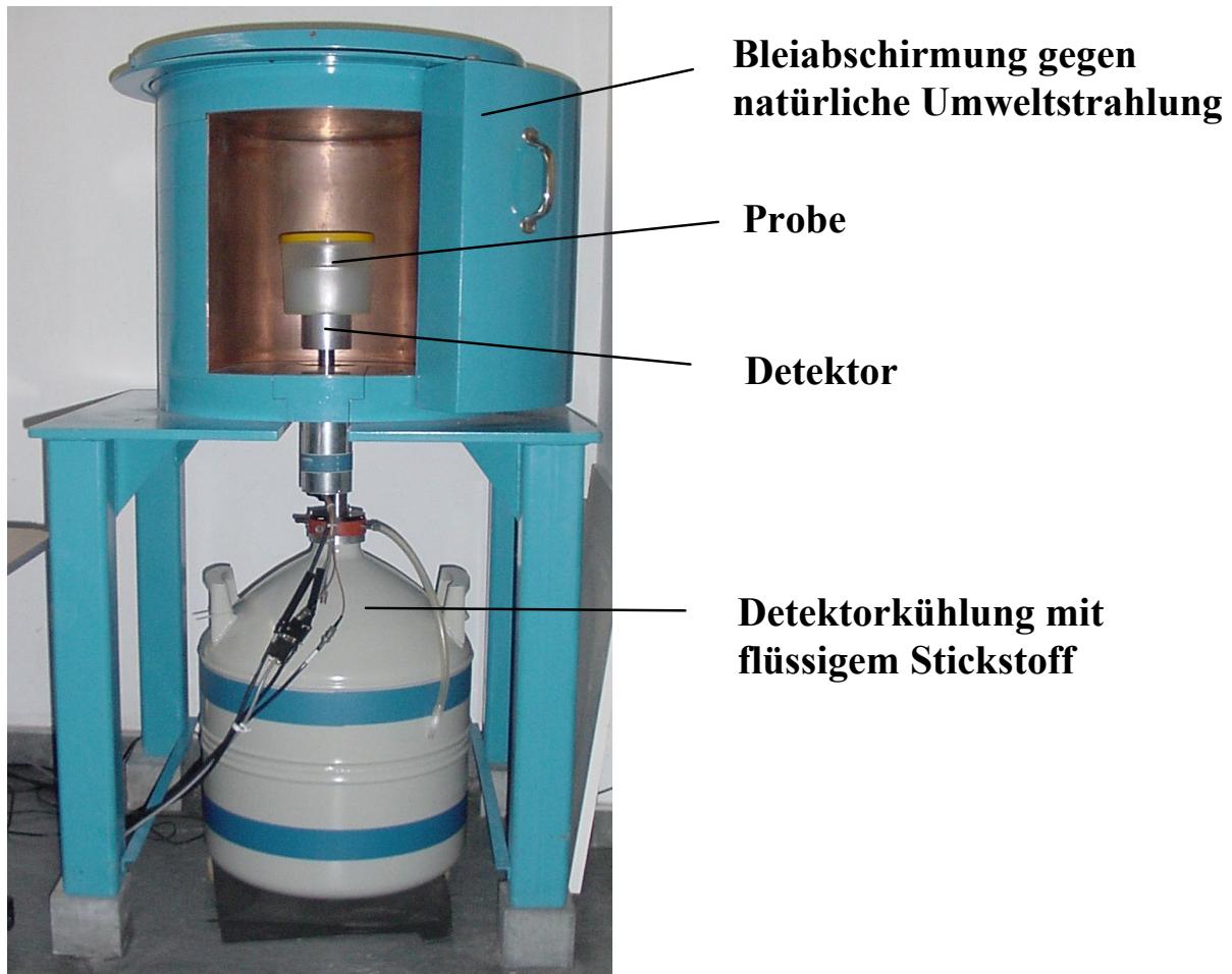
Abbildung 2-6: Messplatz für Gammaspektrometrie: Abschirmung: 1.500 bis 2.000 Kg Blei Probenvolumen: 1 Liter Halbleiter-Detektor: Kristall aus reinstem Germanium mit Verstärker und Vielkanalanalysator Kühlung: 30 L flüssiger Stickstoff
