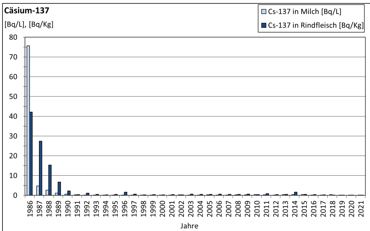
Abbildung 5-3: Jahresmittelwerte von Cs-137 in Milch und Rindfleisch aus NRW von 1986 bis 2021. Im Jahr 2021 wurden insgesamt 104 Milchproben und 55 Rindfleischproben analysiert.
