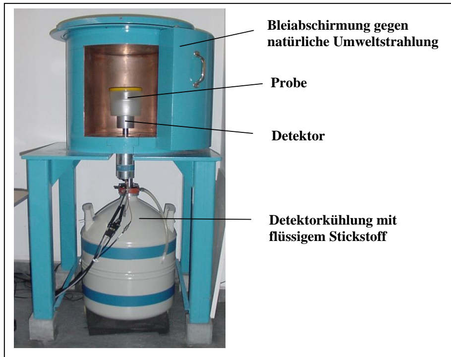
Abbildung 2.6: Messplatz für Gammaskopie: - Abschirmung: 1500 bis 2000 Kg Blei - Probenvolumen: 1 Liter - Halbleiter-Detektor: Kristall aus reinstem Germanium mit Verstärker und Vielkanalanalysator - Kühlung: 30 L flüssiger Stickstoff
