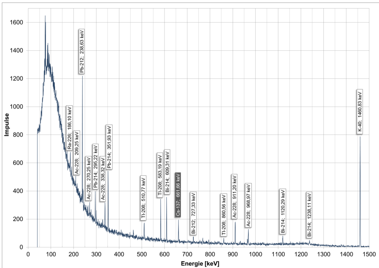
Abbildung 2.5: Gammastrahlungsspektrum mit Energienlinien verschiedener natürlicher Radionuklide sowie des künstlichen Cäsium-137
