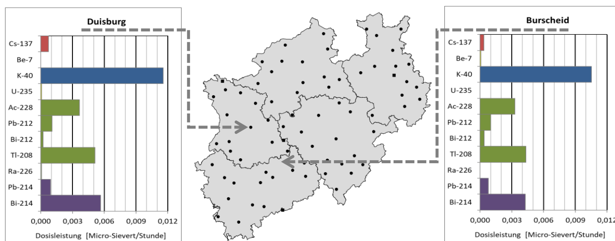
Abbildung 5.7: In-Situ-Gammaspektrometrie in NRW. Die Punkte zeigen die 75 Messstellen verteilt über die fünf Regierungsbezirke. Beispielhaft dargestellt sind Messergebnisse aus dem Jahr 2019 an den Messstellen in Duisburg (05.06.2019) und Burscheid (10.10.2019). Außer Cäsium-137 sind alle gemessenen Radionuklide natürlichen Ursprungs (siehe auch Tabelle 5.3).
