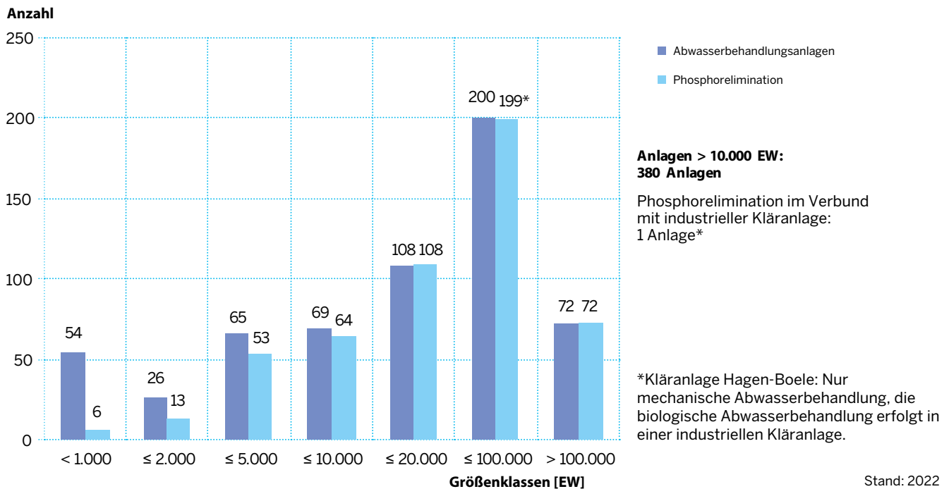
Abbildung 5.4 Kommunale Abwasserbehandlungsanlagen mit chemischer Phosphorelimination
