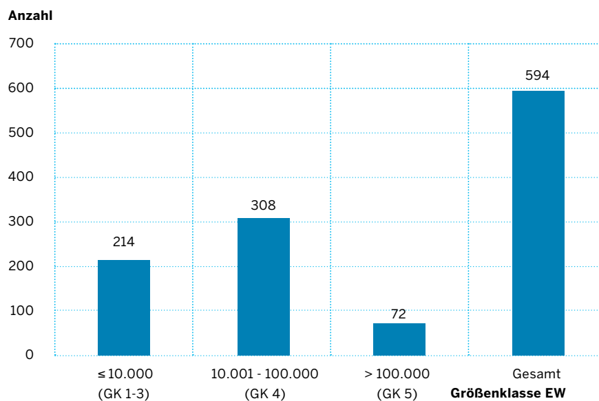
Abbildung 5.1 Anzahl der kommunalen Kläranlagen sortiert nach Größenklassen
