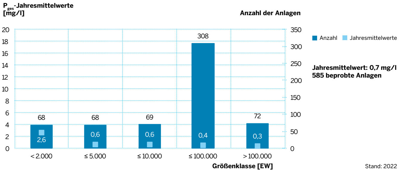
Abbildung 5.9 P_{ges} -Jahresmittelwerte kommunaler Abwasserbehandlungsanlagen aus der amtlichen Überwachung
