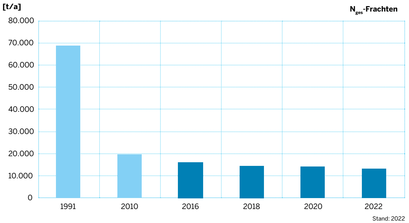
Abbildung 5.15 Entwicklung der Stickstofffrachten aus kommunalen Abwasserbehandlungsanlagen
