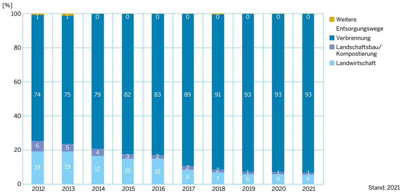
Abbildung 9.3 Entwicklung der Klärschlamm Entsorgung 2012-2021
