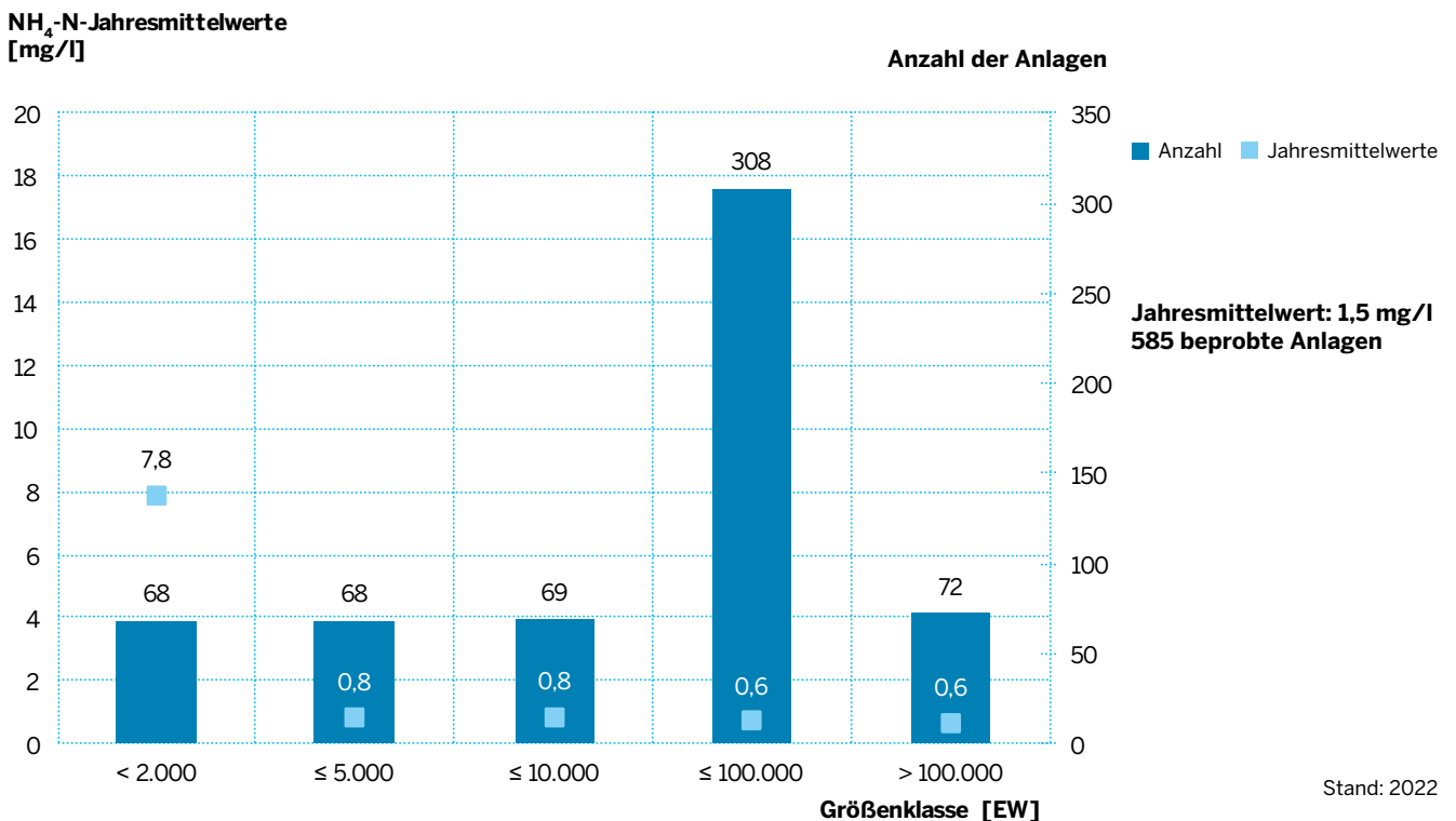
Abbildung 5.6 \text{NH}_4\text{-N} -Jahresmittelwerte kommunaler Abwasserbehandlungsanlagen aus der amtlichen Überwachung
