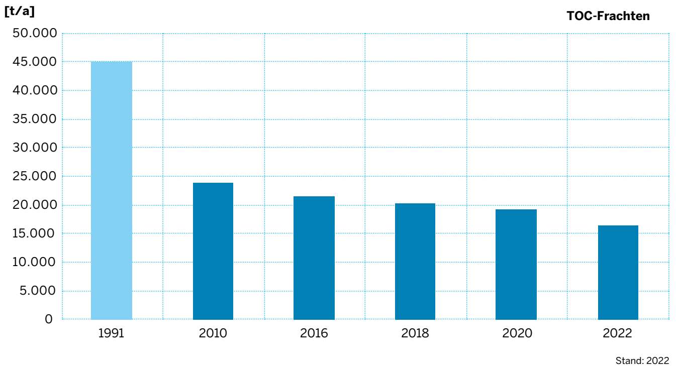
Abbildung 5.14 Entwicklung der TOC-Frachten aus kommunalen Abwasserbehandlungsanlagen
