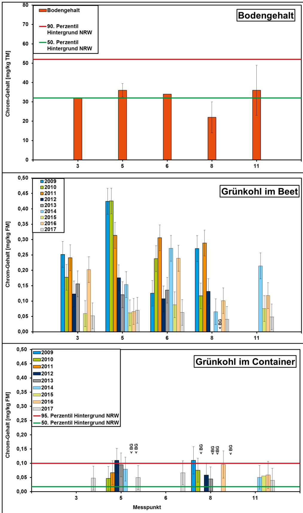
Abbildung 4: Chrom-Gehalte im Boden [mg/kg TM], Grünkohl im Beet und Grünkohl im Container [mg/kg FM; inkl. Standardunsicherheit] an den Messpunkten in Lünen, Hintergrundgehalte in NRW für Boden und Grünkohl
