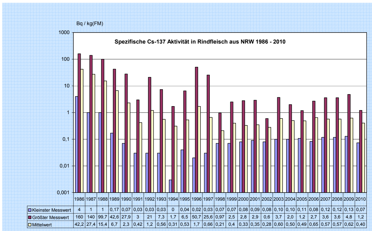
Abbildung 5.4: Spezifische Cs-137 Aktivität in Rindfleisch NRW 1986 - 2010
