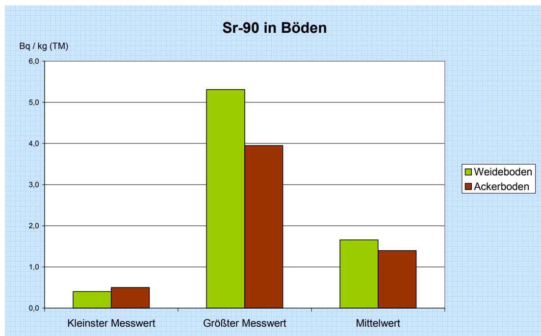
Abbildung 5.2: Spezifische Sr-90 Aktivität in verschiedenen Bodenarten NRW 2010
