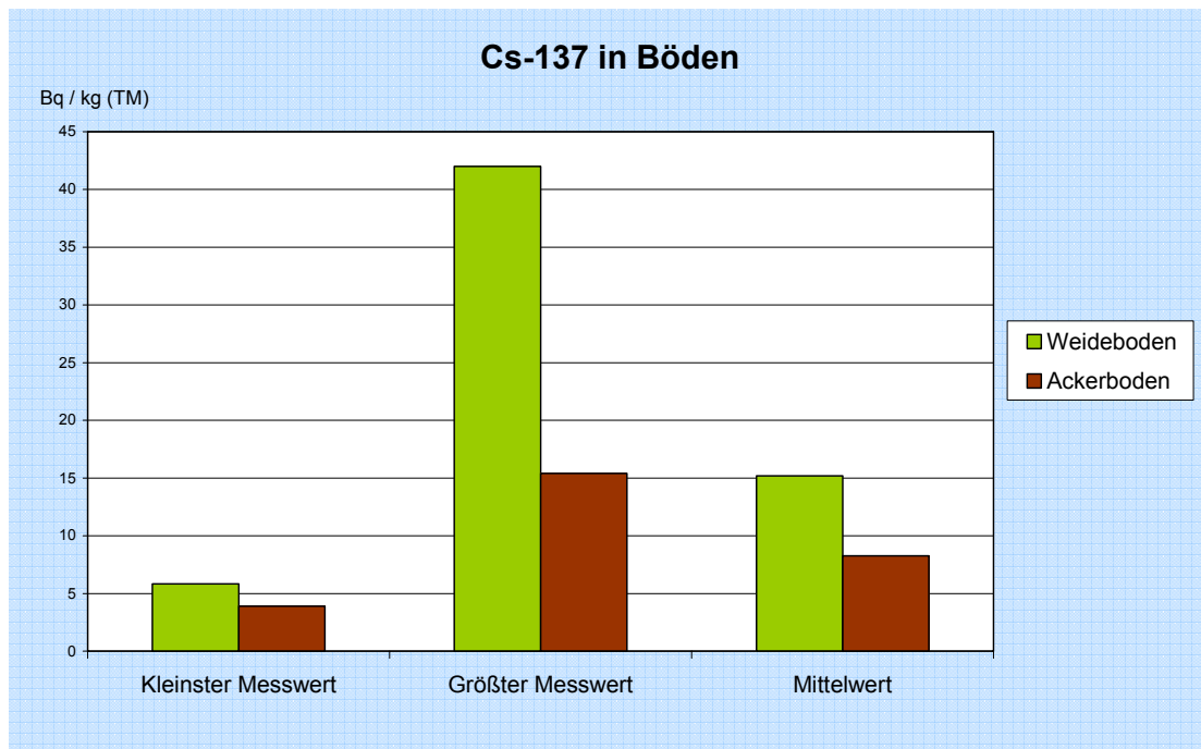
Abbildung 5.1: Spezifische Cs-137 Aktivität in verschiedenen Bodenarten NRW 2010
