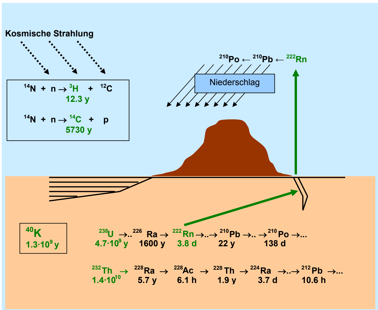
Abbildung 2.3: Natürliche radioaktive Stoffe in Atmosphäre und Boden und deren physikalische Halbwertszeiten (y = Jahre, d = Tage, h = Stunden, 10^9 = 1 Milliarde)
