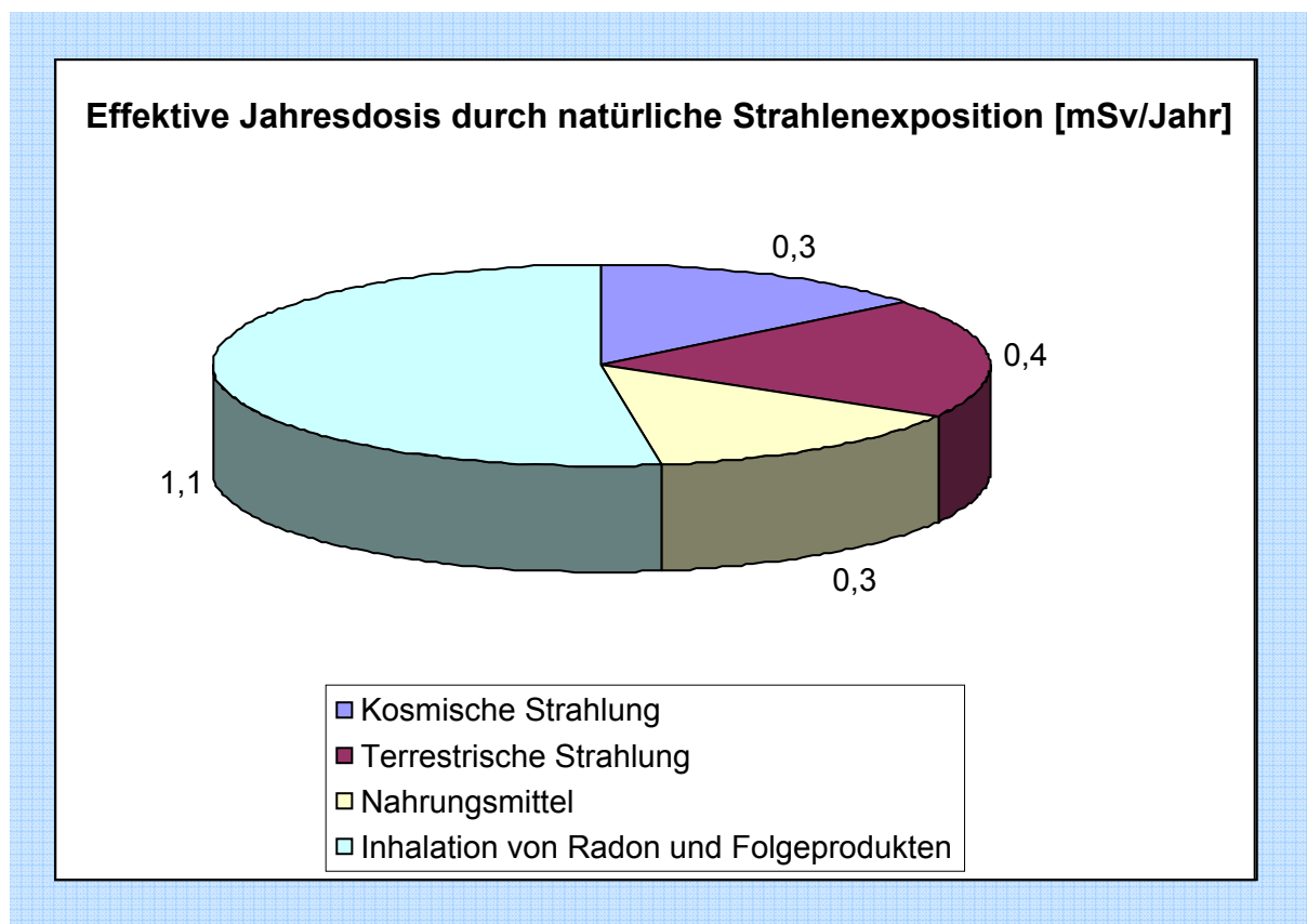
Abbildung 2.4: Zusammensetzung der mittleren effektiven Jahresdosis durch natürliche Strahlenexposition
