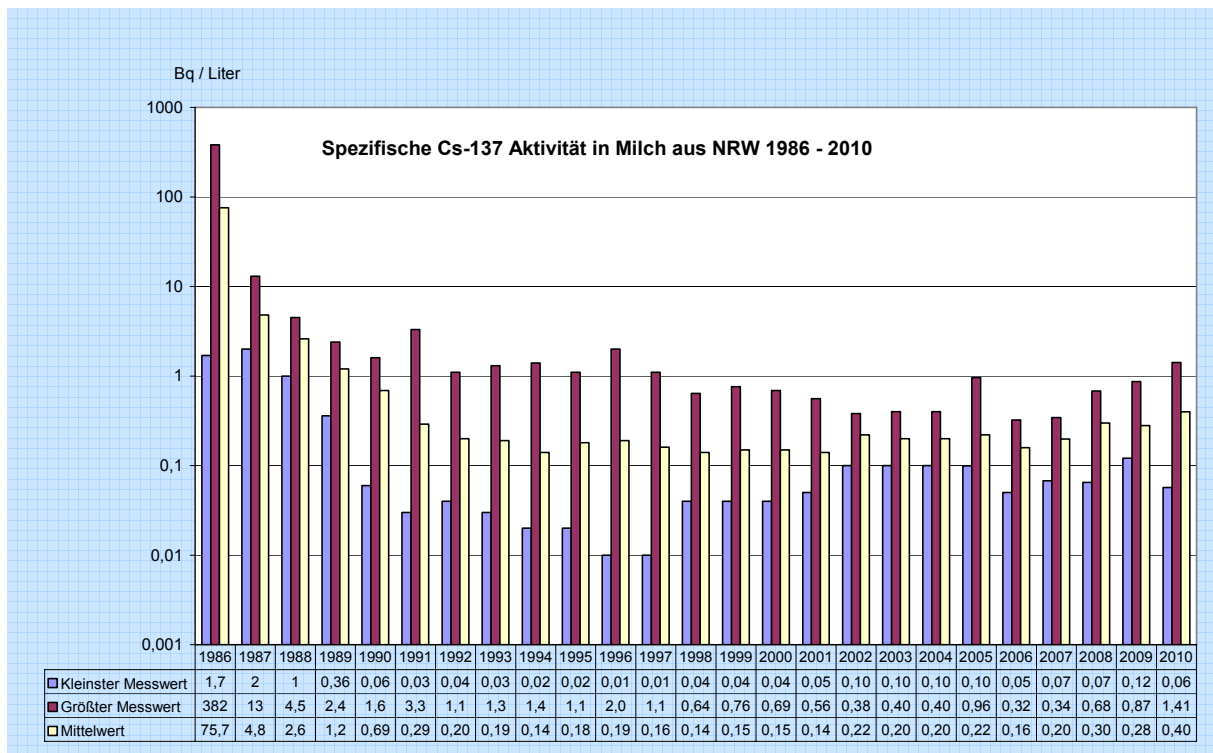
Abbildung 5.3: Spezifische Cs-137 Aktivität in Milch NRW 1986 - 2010
