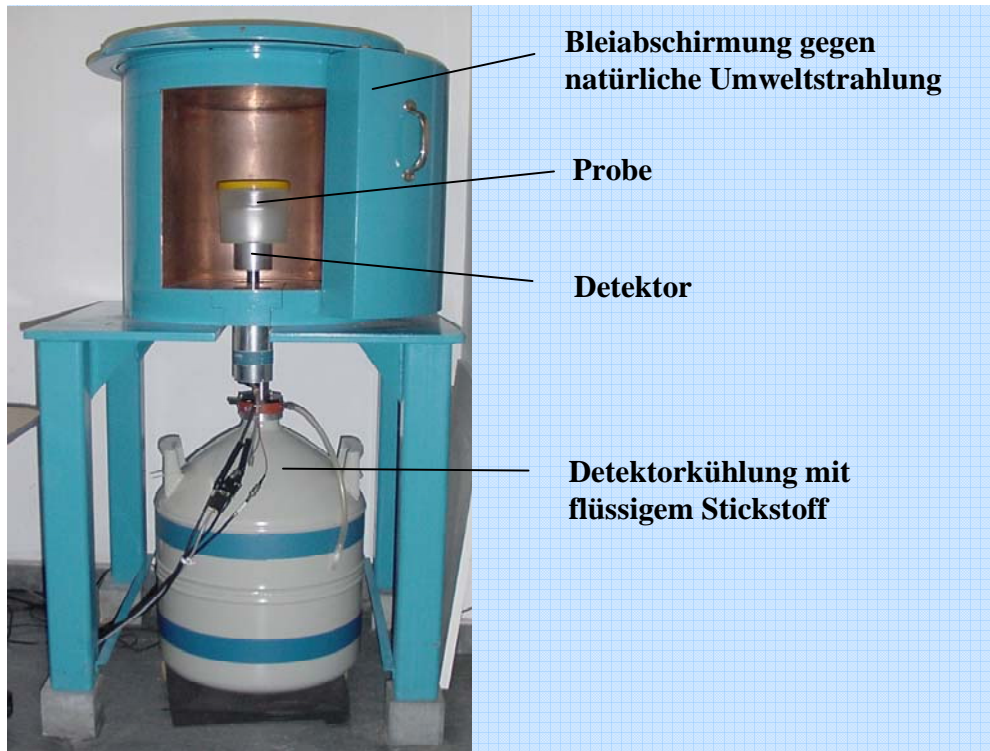
Abbildung 2.5: Messplatz für Gammaskpektrometrie
