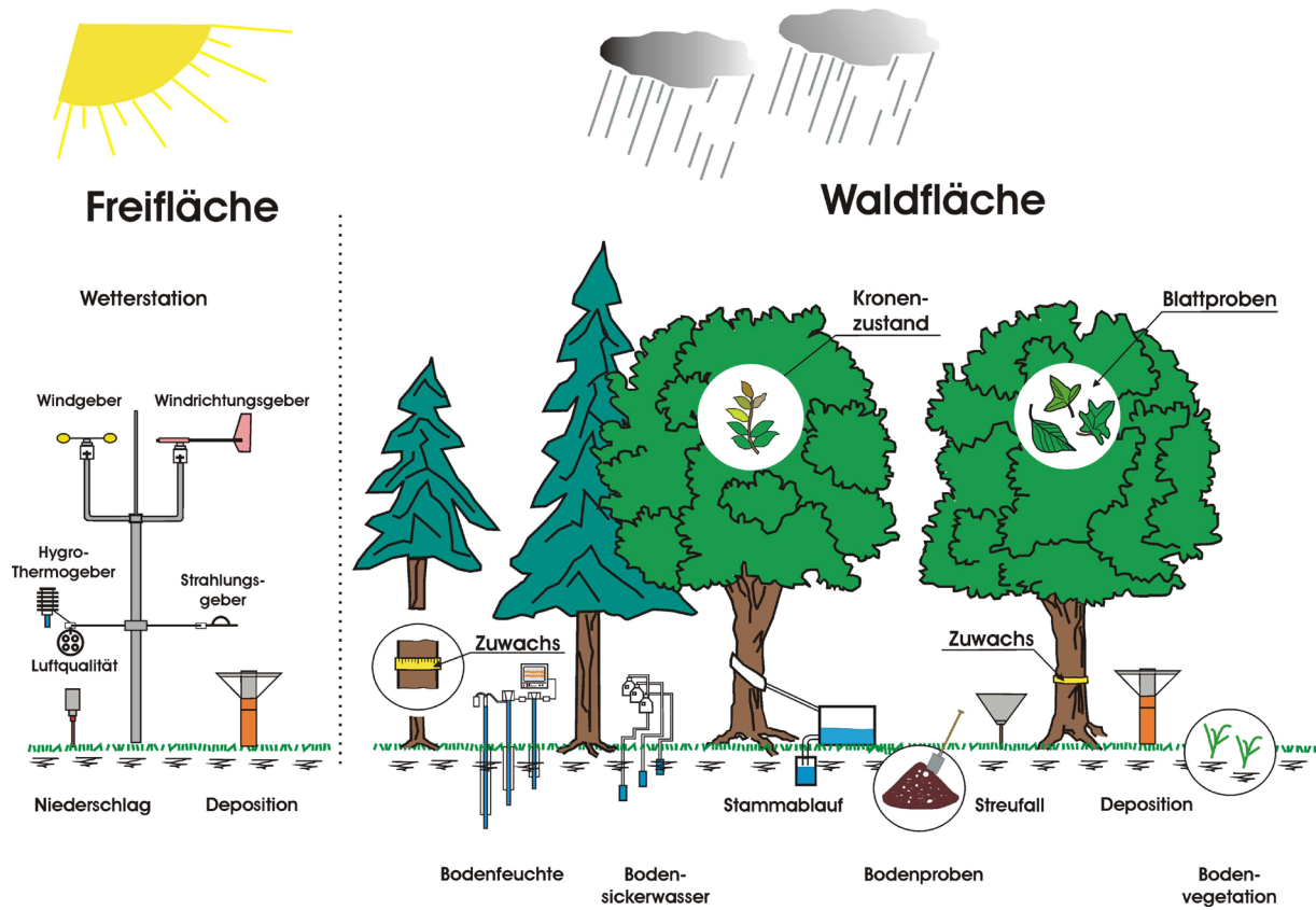
Abb. 4 (Schema IM-Fläche): Schematischer Aufbau und Erhebungsparameter auf einer Level-II-Kernfläche des intensiven forstlichen Umweltmonitorings (© Ralf-Michael Büscher).
